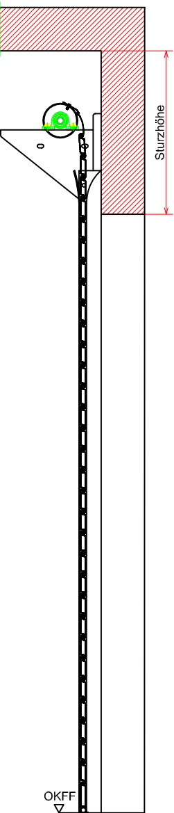
Schnitt B-B
